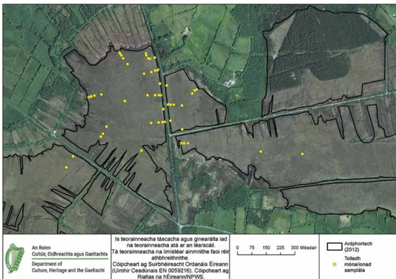
Léaráid A4.11: Ionaid na bpointí samplála móna ar Phortach Chill Taobhain agus sa réimse cóngarach dó, Limistéar SAC Loch Rí, Co. Ros Comáin.
