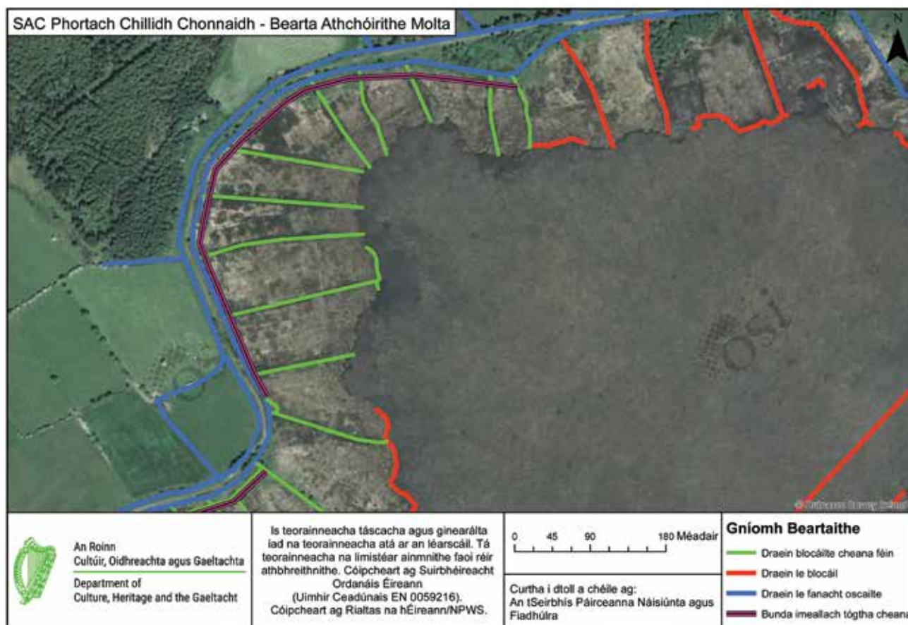
Léaráid 4.1: Mapa ar a léirítear an obair athchóiriúcháin atá beartaithe maidir le réimse de Limistéar SAC Phortach Choill Chonnaidh, Co. an Chabháin/Co. na Mí
