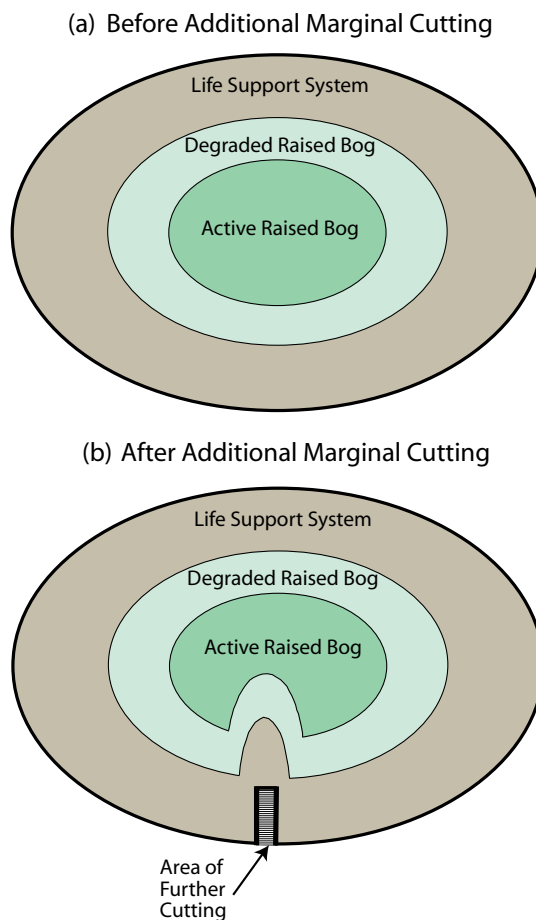
Léaráid 2.4: Scéimléaráid maidir leis an tionchar díréireach is féidir a theacht ar ghnáthóg portaigh ardaithe beo agus díghrádaithe de bharr móin a bhaint i réimse atá ina “thaca beatha”
