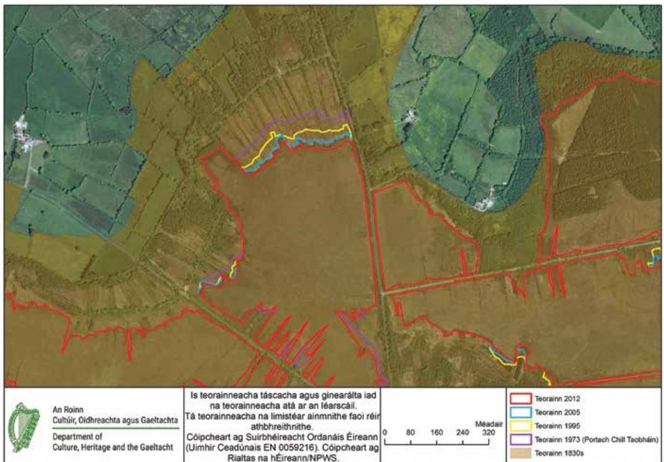
Léaráid A4.4: Imeall neamhbhearnaithe Phortach Chill Taobháin, de réir na mapála a rinne an tSuirbhéireacht Ordanáis sa bhliain 1838 (faoi dhath donn), á leagan anuas ar theorainneacha na láithreach mar a bhí sna blianta 1973, 1995, 2005 agus 2012 (sonraí de chuid OSI agus GSI).
