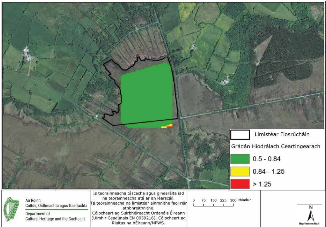
Léaráid A4.21: Mapa ar a léirítear na fánáin hiodrálach measta ingearacha ar fud Phortach Chill Taobháin. Ní sháraítear fánáin chriticiúla thar an limistéar a bhfuil sé beartaithe móin a bhaint ann agus mar sin níltear ag súil le tionchar hidrigeolaíoch
