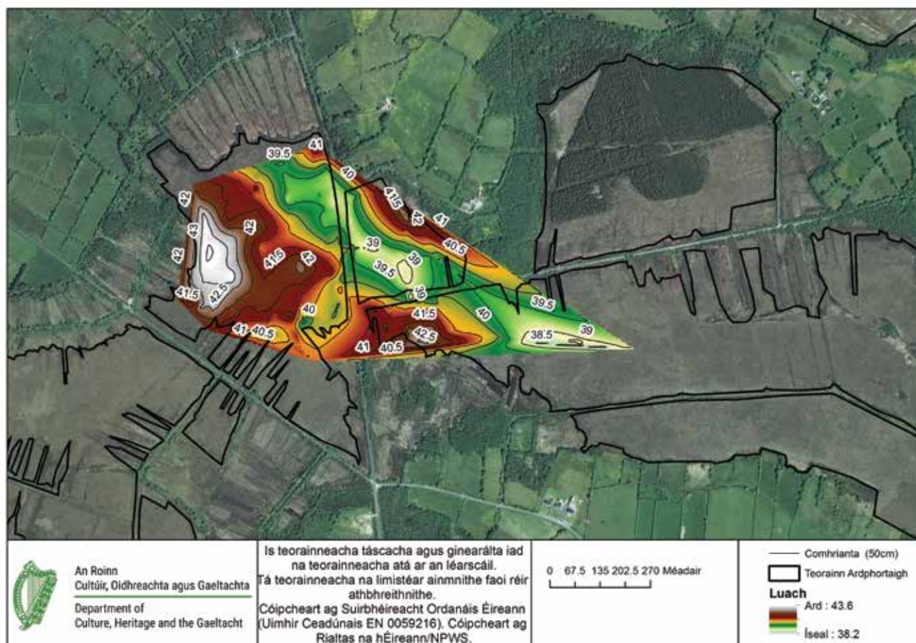
Léaráid A4.13: Mapa dromchla fhoshraith móna de Phortach Chill Taobháin agus an limistéar díreach soir uaidh, ag teannadh leis na réimsí is cóngaraí de phortach DRB, Limistéar SAC Loch Rí.
