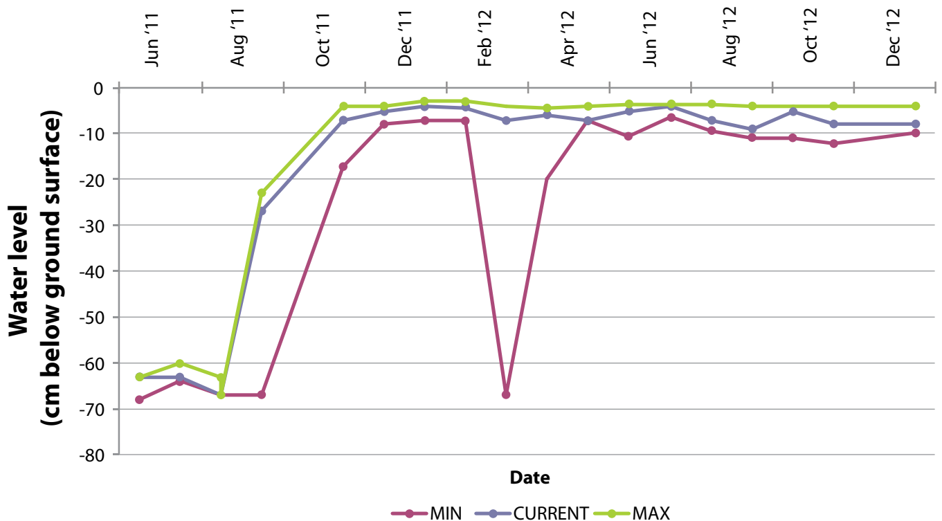
Tábla 4.4: Ardú suntasach maidir leis an maoschlár a tugadh chun aire ag písimeádar uimh. 6 ar Phortach na Greallaí, Co. na Mí, mar gheall ar ghlanleagan na gcrann buaircíneach i mí Lúnasa 2011 (mar chuid de na bearta athchóiriúcháin faoi Thionscadal LIFE Choillte)
