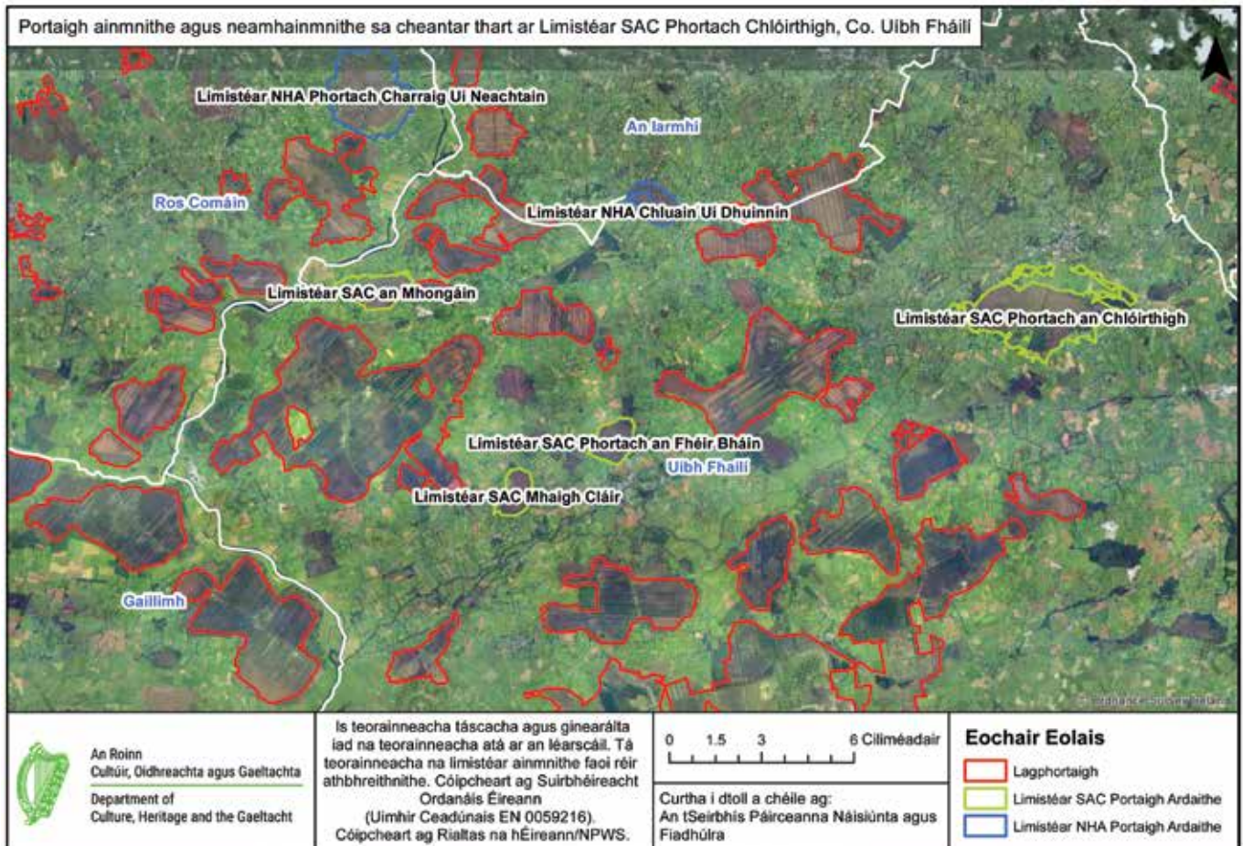
Léaráid 2.3: Portaigh ainmnithe agus neamhainmnithe sa cheantar thart ar Limistéar SAC Phortach Chlóirtheigh, Co. Uíbh Fháilí
