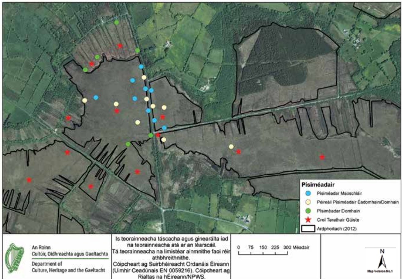
Léaráid A4.12: Ionaid na bpísimeádar agus pointí samplála tarathar gúiste ar Phortach Chill Taobháin agus sa réimse cóngarach dó, Limistéar SAC Loch Rí
