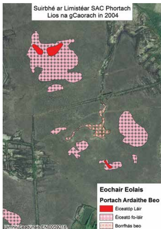
Léaráid 4.2: Limistéar SAC Phortach Ardaithe Lios na gCaorach, Co. na Gaillimhe. Sampla d'obair athchóiriúcháin le dambaí móna ar phortach ard a raibh dea-thoradh uirthi. Is léiriú fairsingiú ar an réimse dearg (éiceatóp láir) agus ar an réimse bándearg (fo-réimse láir) ar an méadú a tháinig ar phortach ardaithe beo mar gheall ar an obair athchóiriúcháin
