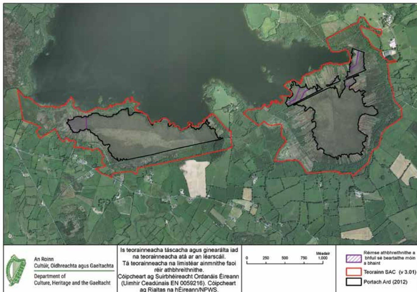
Léaráid 5.3: Réimsí taobh istigh de Phortach Mhuine Bheag agus de Phortach Dhoire Mhic Aogáin inar féidir móin a bhaint gan cur isteach ar aidhmeanna caomhantais sonracha maidir le portach ardaithe beo ar an láthair
