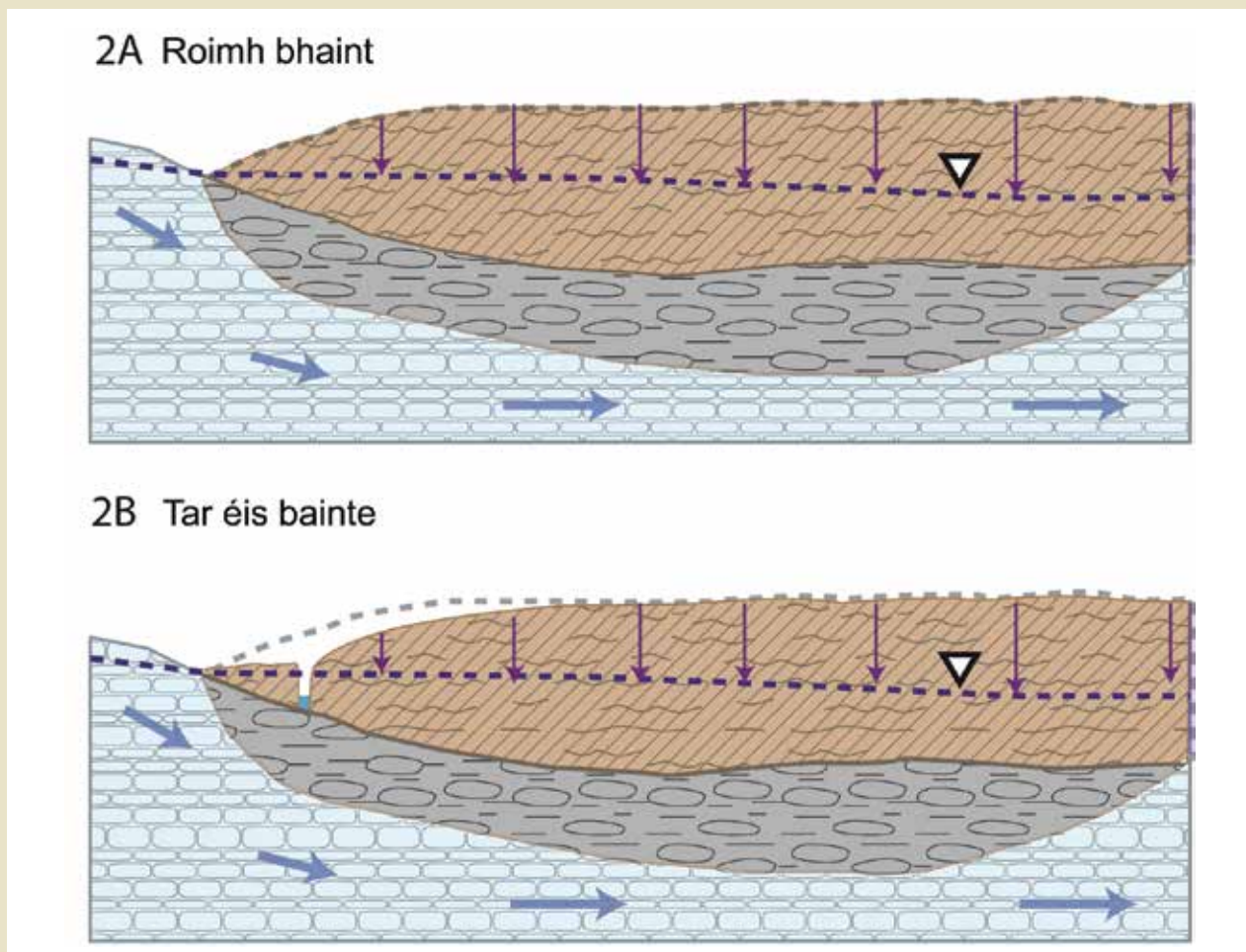
Léaráid A4.20: Léiriú ar an gcosaint a thugann foshraith ar bheagán tréscailteachta (faoi dhath dorcha liath) d'uiscíoch faoi bhun portaigh móna ar an tionchar a bheadh ag draenáil imeallach. Síneann tionchar eicihiodreolaíocha ar an bportach chuig limistéar níos lú áit nach bhfuil tionchar ar an réimeas srutha screamhuisce san uiscíoch faoina bhun.
