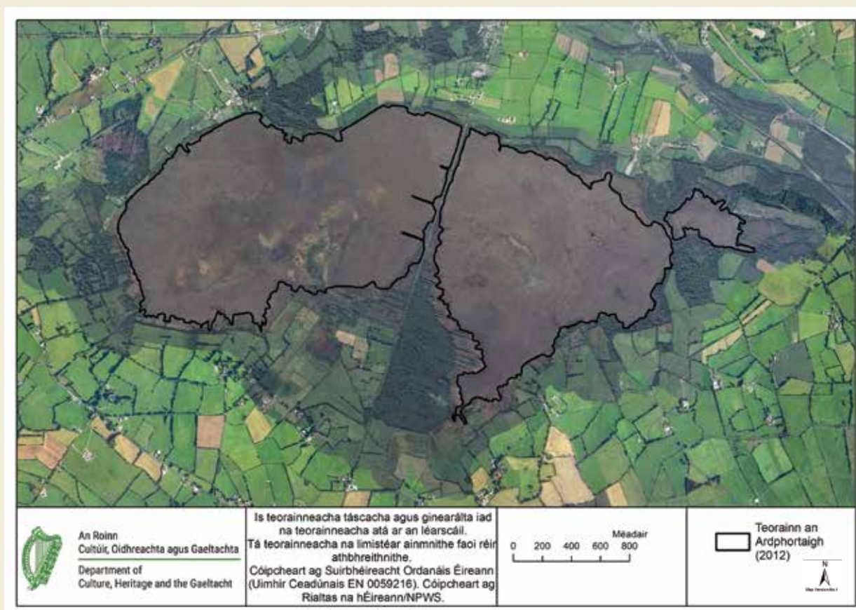
Léaráid A2.2:SAC Phortach Chlóirthigh, Co. Uíbh Fhailí, grianghraf ón aer atá curtha ina ceart go geoiméadrach a thaispeánann teorainn an phortaigh ardaithe
