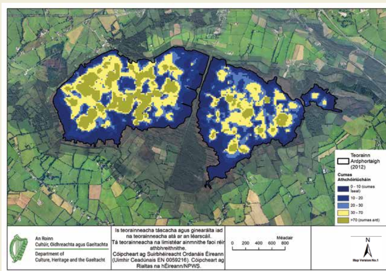
Léaráid A2.7:SAC Phortach Chlóirithigh, Co. Uíbh Fhailí, cumas athchóiriúcháin faighte ón tsamhail eicihidreolaíoch
