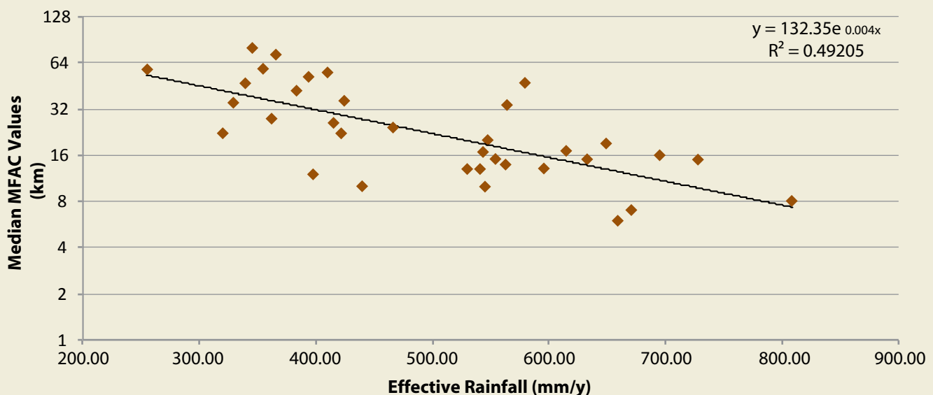
Léaráid A2.1: An gaol idir an meán MFAC agus báisteach
