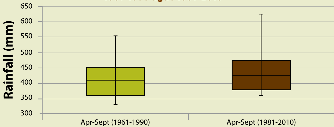
Léaráid 2.6: Codarsnacht maidir le báisteach i rith an tsamhraidh ar fud na tíre (Aib.-M.F.)
