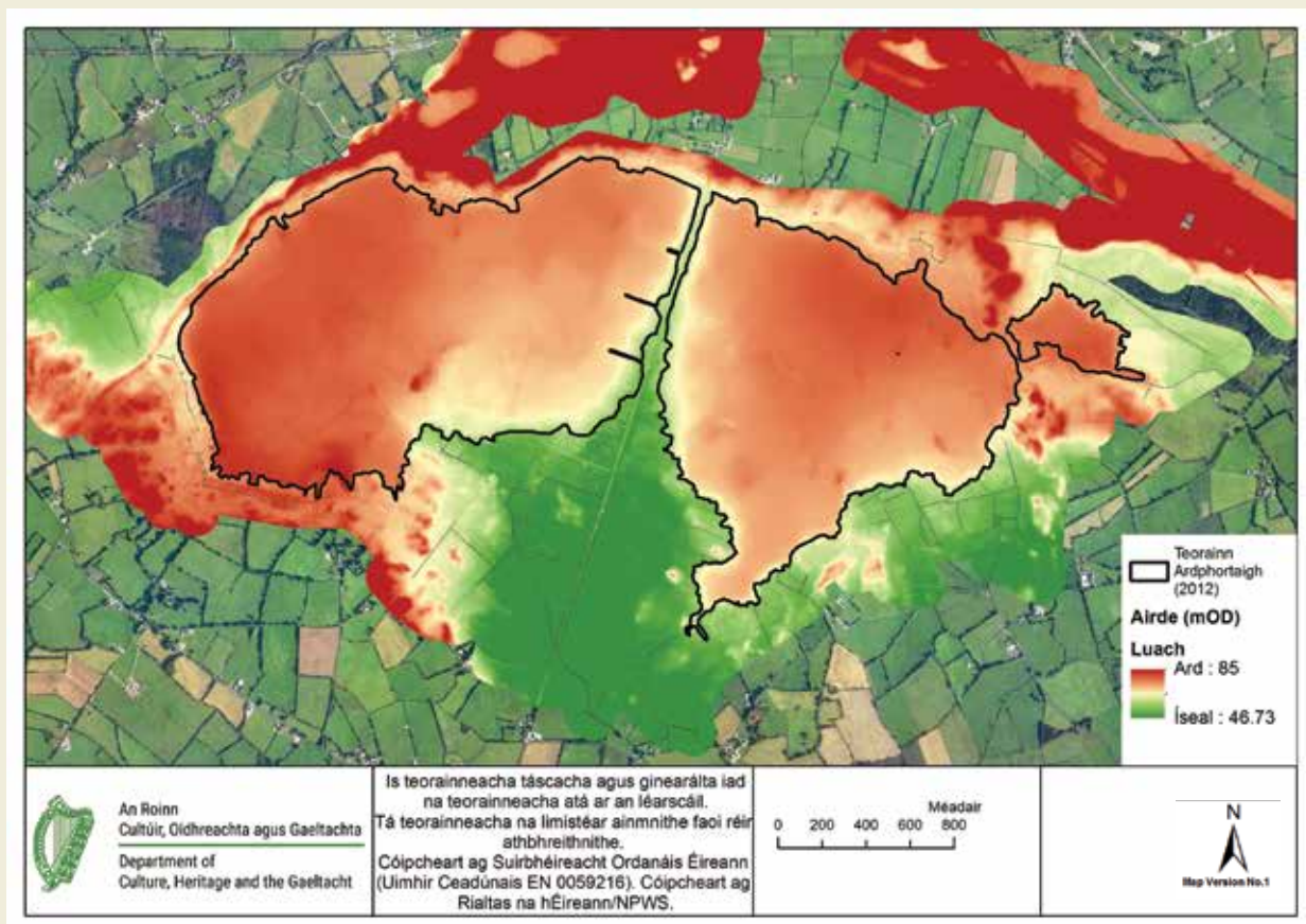
Léaráid A2.4:SAC Phortach Chlóirthigh, Co. Uíbh Fhailí, íomhánna LiDAR 2012
