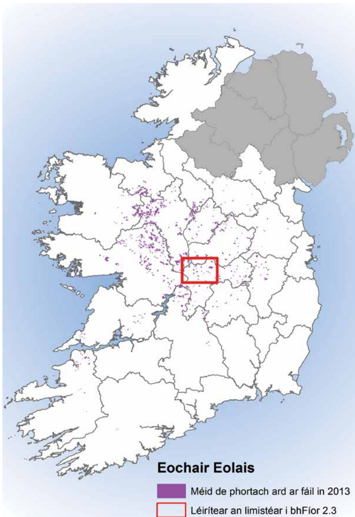
Léaráid 2.2: Mapa ar a léirítear an méid den phortach ard atá ar fáil go fóill i bPoblacht na hÉireann
