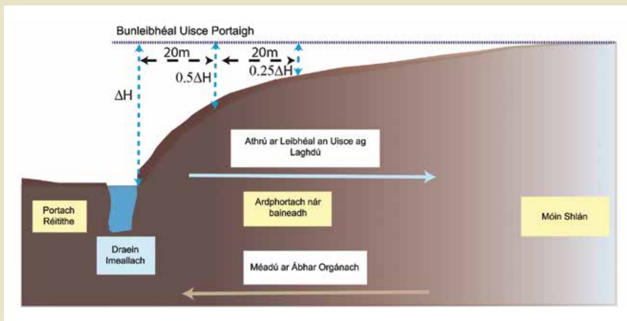
Léaráid A4.17: Scéimléaráid lena léirítear an tionchar a bhíonn ag draenáil móna ar leibhéal uisce agus ar an ábhar orgánach.
