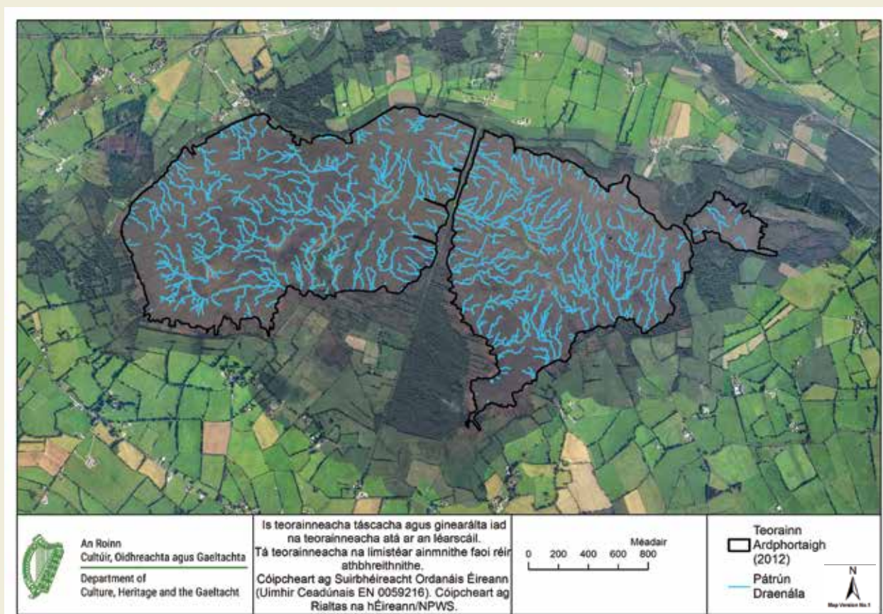
Léaráid A2.6:SAC Phortach Chlóirithigh, Co. Uíbh Fhailí, slite draenála faighte ó íomhánna LiDAR 2012
