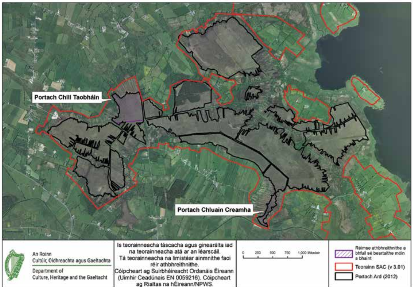
Léaráid 5.2: Réimsí taobh istigh de Limistéar SAC Loch Rí inar féidir móin a bhaint gan cur isteach ar aidhmeanna caomhantaí sonraigh maidir le portach ardaíthe beo ar an láthair
