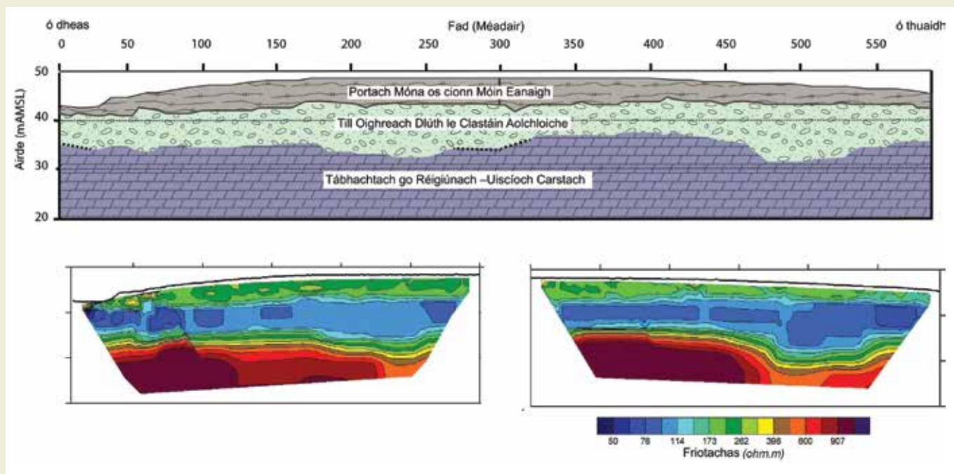
Léaráid A4.14: Trasghearradh geolaíochta arna ríomh de réir sonraí geofisice agus geolaíochta le traschrios ERT R4 ar Phortach Chill Taobháin; (Thíos) Torthaí Suirbhéireacht ERT maidir le traschrios ERT R4, Portach Chill Taobháin, Limistéar SAC Loch Rí. Tabhair ar airdtíús suntasach an ábhair fhoshraithe faoi bhun na móna (till oighreach dlúth le clastáin aolchoilche)
