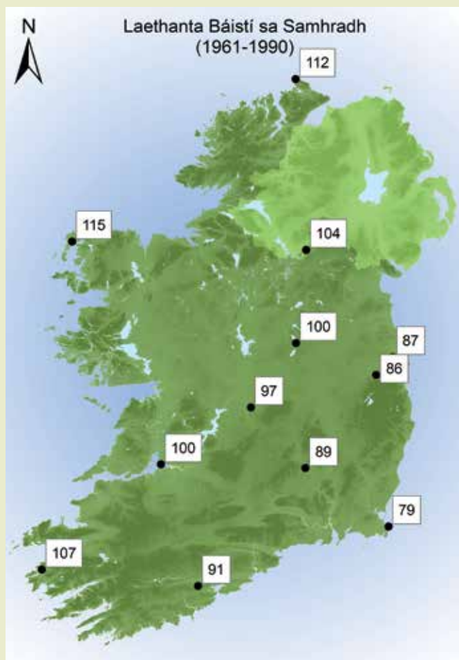
Léaráid 2.7: Codarsnacht maidir le laethanta báistí i rith an tsamhraidh ar fud na tíre
